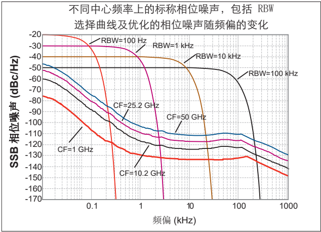
图3. 选件035不同中心频率处的额定相位噪声
